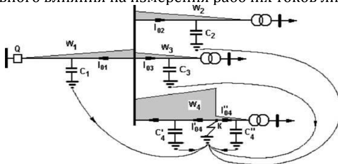
Рис. 1. Схема сети и эюры показаний переносного прибора в различных ее участках
